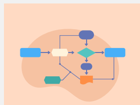
Flussdiagrammerstellung
